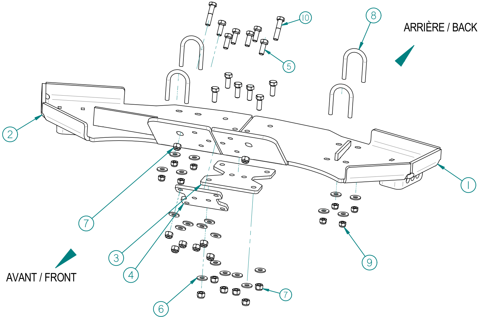
Liste des pièces / Part List
