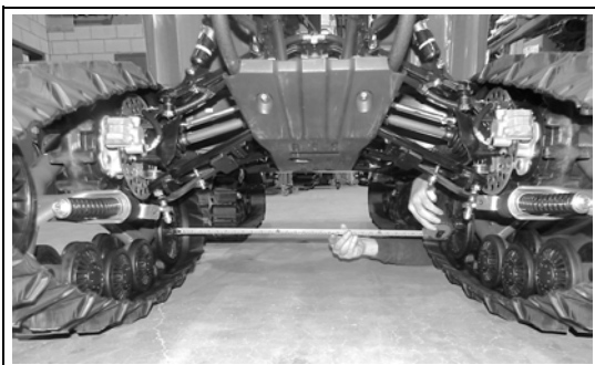
Figure 23 (Distance entre les roues arrière)
